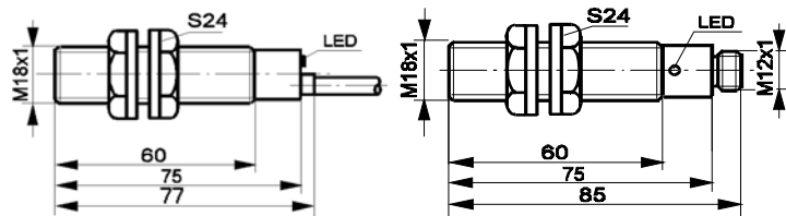
wyjście kablowe
