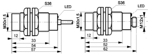
wyjście kablowe
