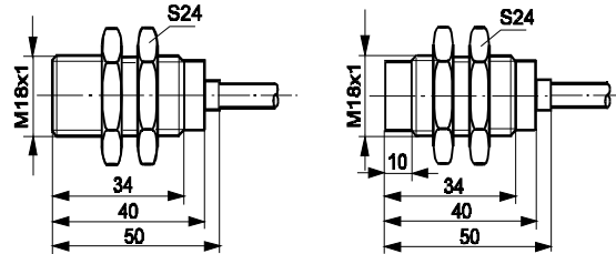
Czoło wbudowane
