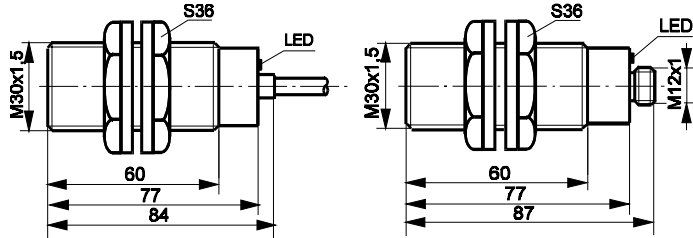
wyjście kablowe
