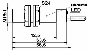
wyjście kablowe
