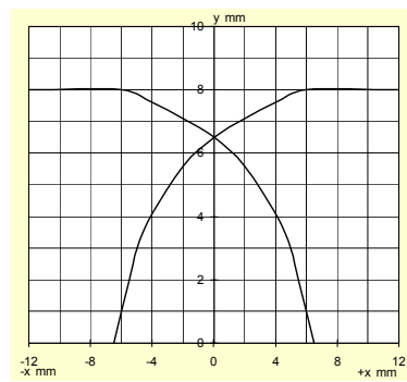
Response characteristics/Ansprechkennlinie:
