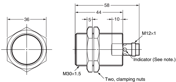
E2A-M30KS15-M1-□□/E2A-S30KS15-M1-□
